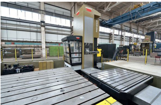
CNC MILLING MACHINING - TOS VARNSDORF WHQ13 AND WRD15
